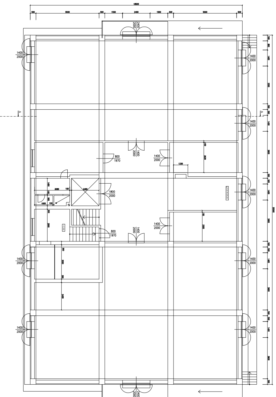
PŮDORYS 1.NP - SKLAD č. 29
